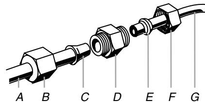
A. Conduit vers le réfrigérateur B. Écrou (fourni) C. Raccord D. Raccord (à acheter) E. Virole (à acheter) F. Écrou (à acheter) G. Canalisation d'eau du domicile
